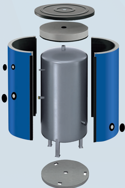
Snímatelná izolace
